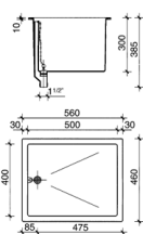
Мойка из полипропилена врезная (560×460×385)
