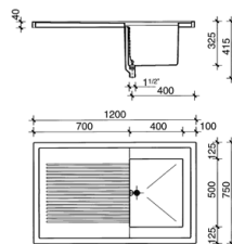
Мойка из полипропилена накладная одинарная (1200×750×415)
