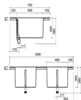
Мойка из полипропилена двойная врезная (1200×750×385)
